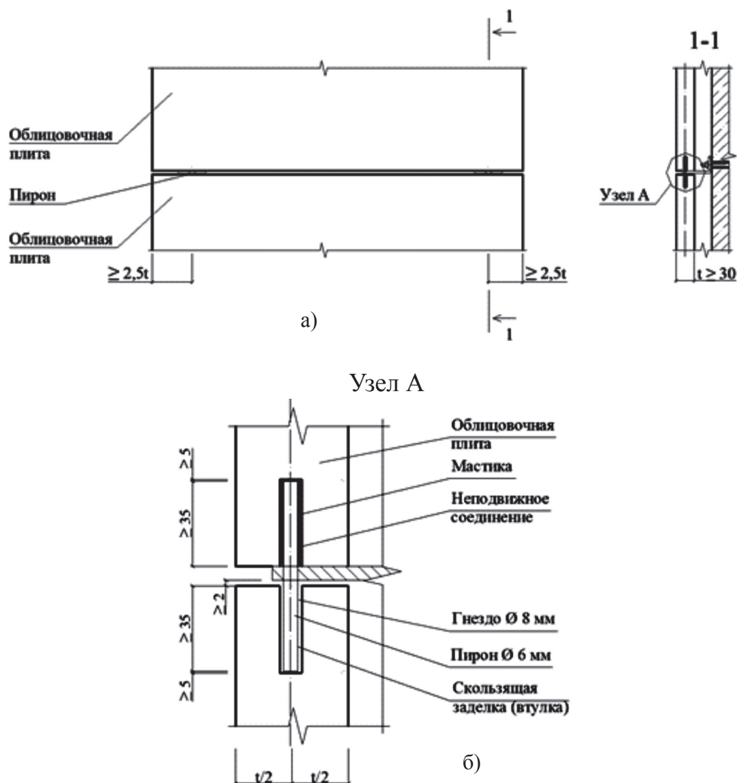
а) общий вид; б) вариант установки пилона
