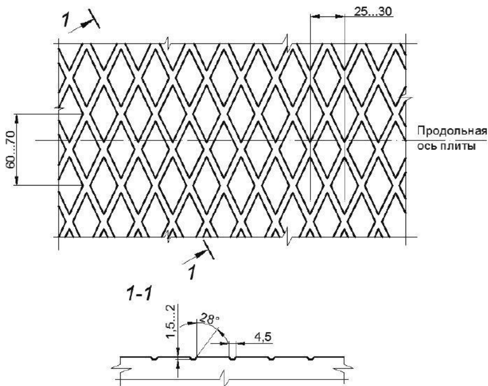
Рисунок 2 - Фрагмент рифления рабочей поверхности плиты
