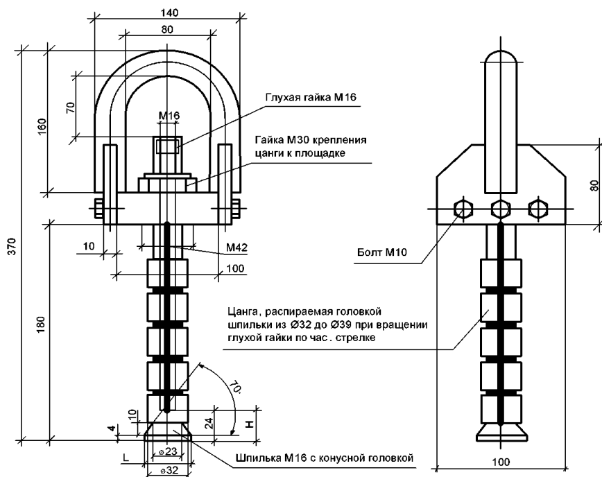
Рисунок А.4 - Вариант конструкции цангового захвата
