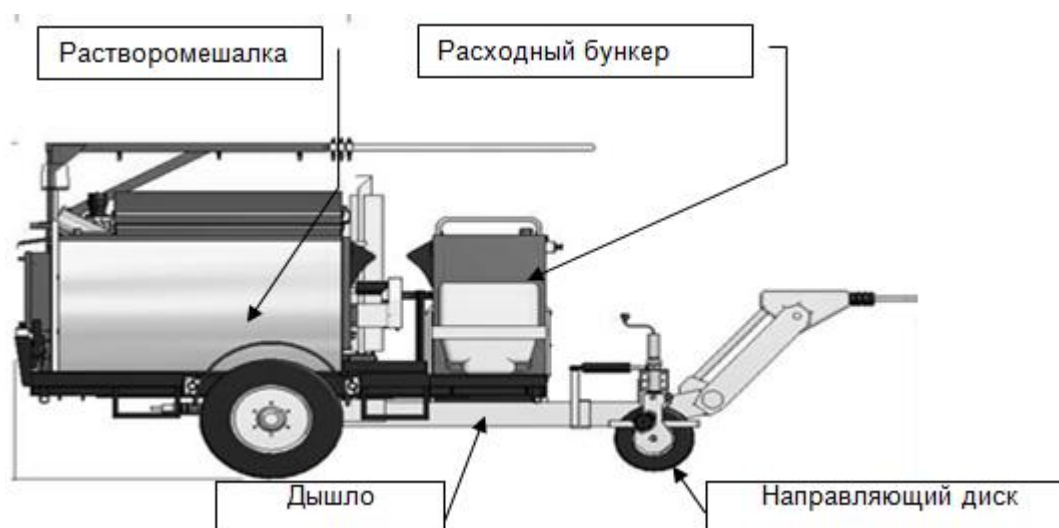
Рисунок 13 - Вариант конструкции заливщика шва
