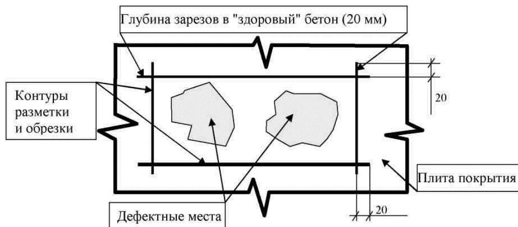
Рисунок 15 - Вариант схемы разметки и нарезки на покрытии дефектных мест
