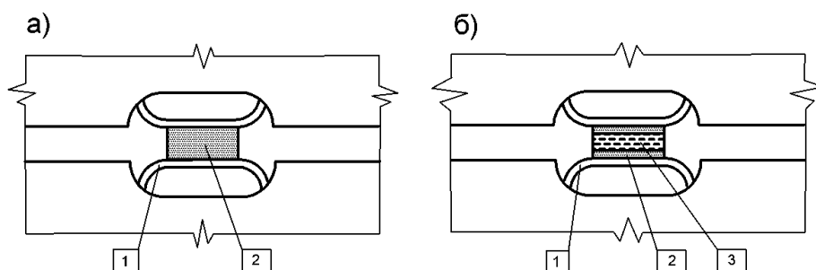
1 - стыковая скоба; 2 - сварной шов; 3 - дополнительный стержень а - при зазоре до 4 мм; б - при зазоре между скобами более 4 мм
