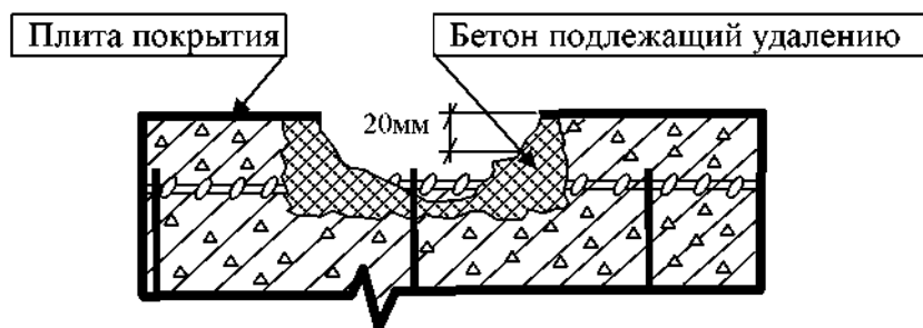
Рисунок 16 - Вариант схемы удаления поврежденного бетона на покрытии
