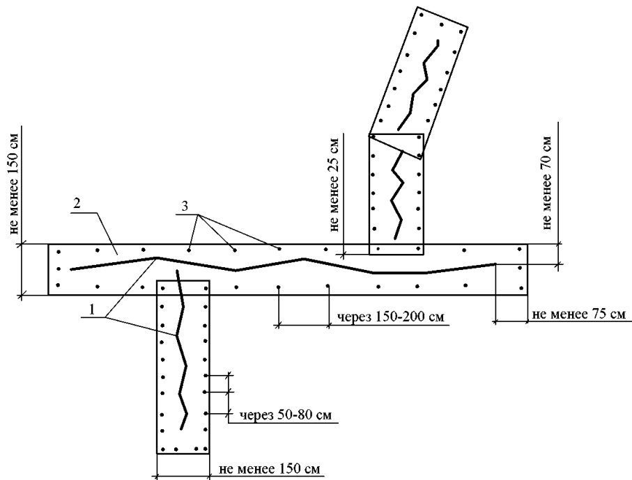
Рисунок 19 - Вариант сплошной укладки и крепления трещинопрерывающей (армирующей) прослойки на кривых малого радиуса
