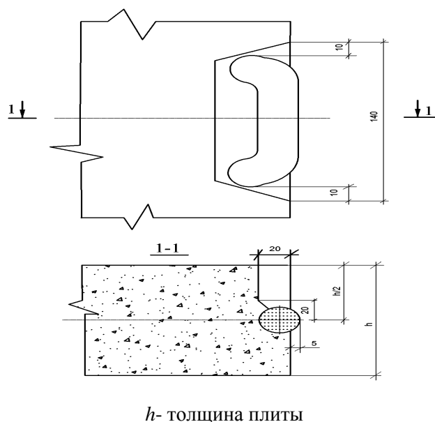
Рисунок А.2 - Вариант конструкции стыкового соединения
