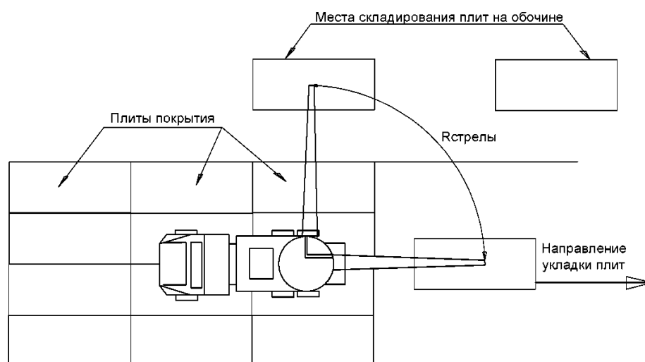
Рисунок 4 - Схема складирования плит на обочине
