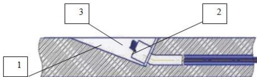
1- крепежный карман, 2 – анкер, 3 – обрезанный стальной канат
