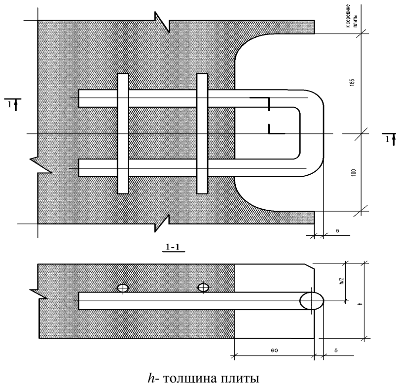
Рисунок А.1 - Вариант конструкции монтажно-стыкового соединения
