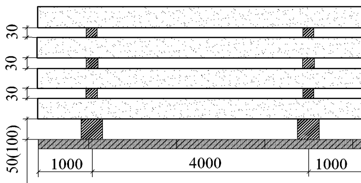
Рисунок 3 - Схема складирования плит
