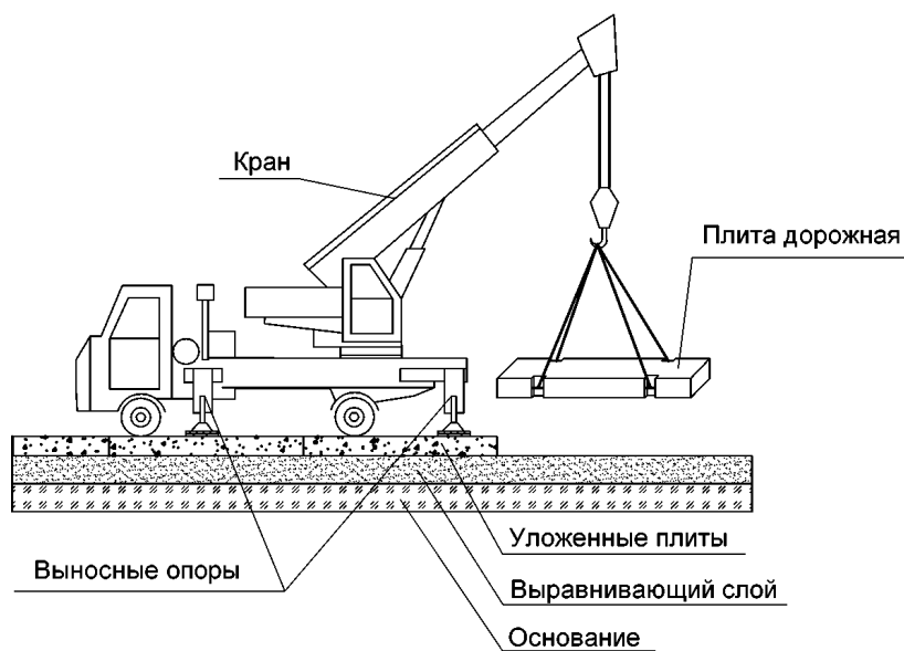
Рисунок 7 - Укладка плит краном с установкой выносных опор
