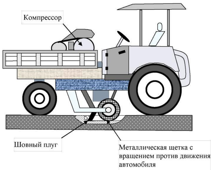
Рисунок 14 - Вариант щеточной машины оборудованной шовным плугом
