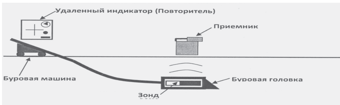
Рисунок В.2 – Схема действия электромагнитной системы подземной локации
