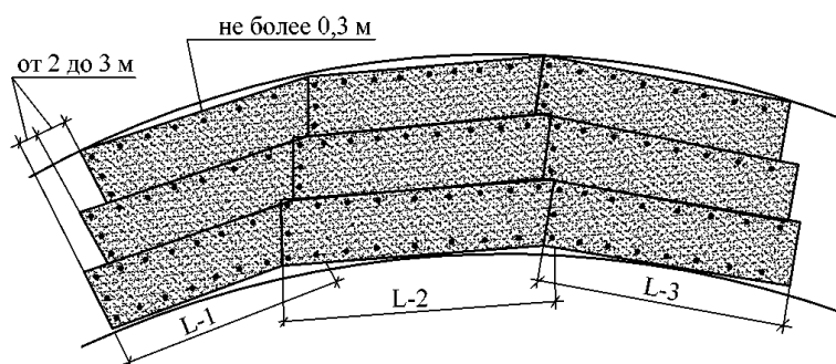
Рисунок 18 - Вариант сплошной укладки и крепления трещинопрерывающей (армирующей) прослойки на кривых малого радиуса
