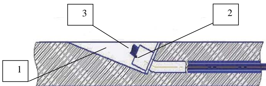
1- крепежный карман, 2 – анкер, 3 – обрезанный стальной канат
