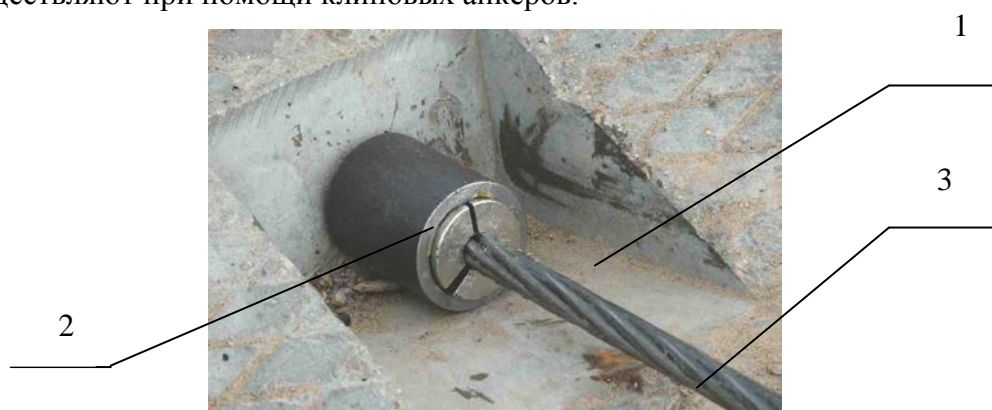
1 – крепежный карман, 2 – анкер, 3 – стальной канат
