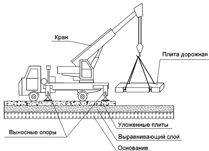
Рисунок 6 - Укладка плит краном с установкой выносных опор
