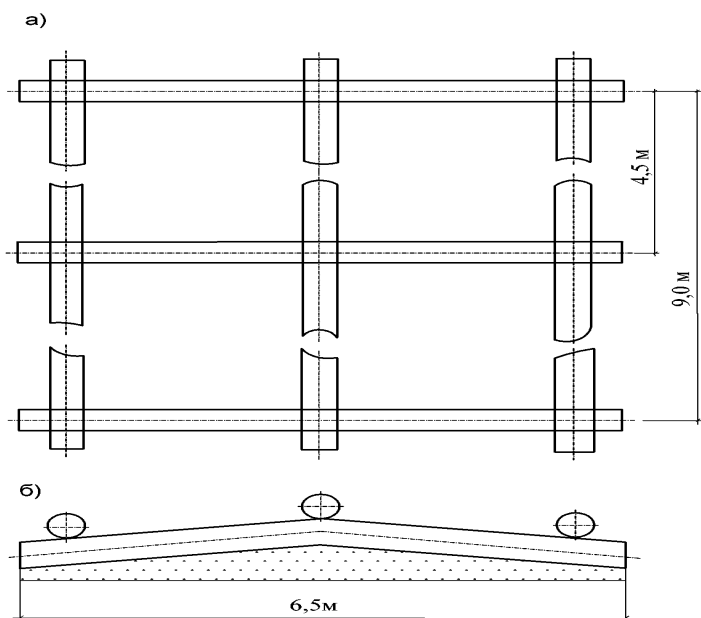
а - вид сверху; б - вид спереди
