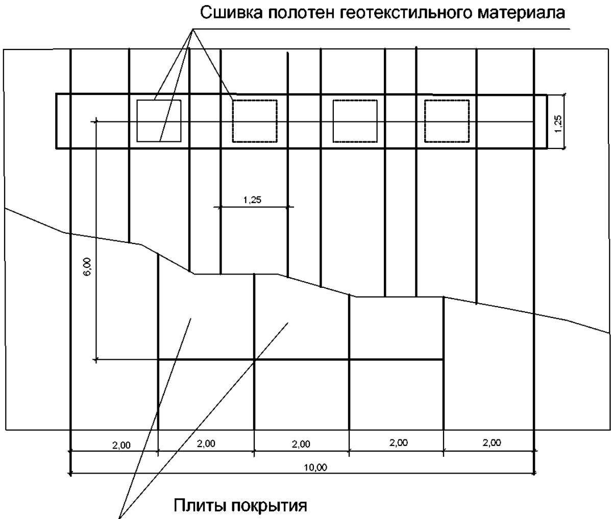
Рисунок 10 - Вариант раскладки геотекстильного материала полосами под швами и кромками покрытия
