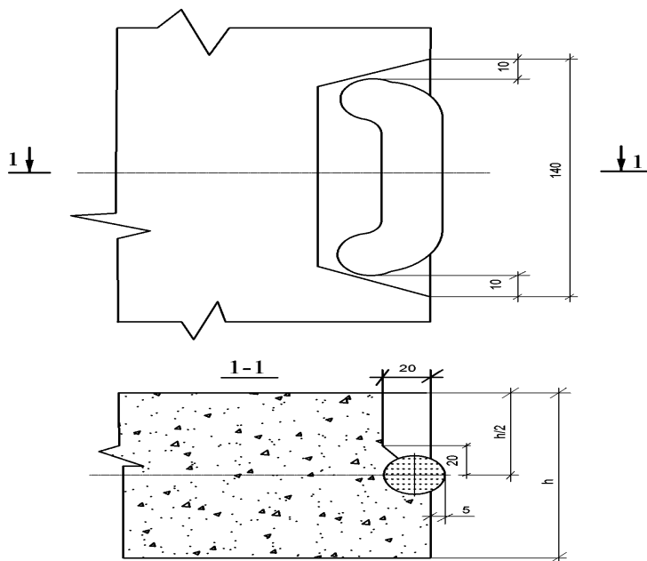
Рисунок А.2 - Вариант конструкции стыкового соединения
