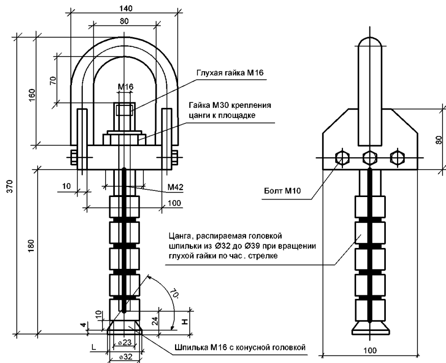
Рисунок А4 - Вариант конструкции цангового захвата
