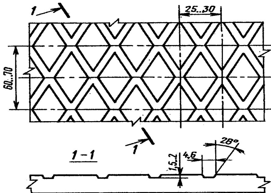
Рисунок 2 - Фрагмент рифления рабочей поверхности плиты
