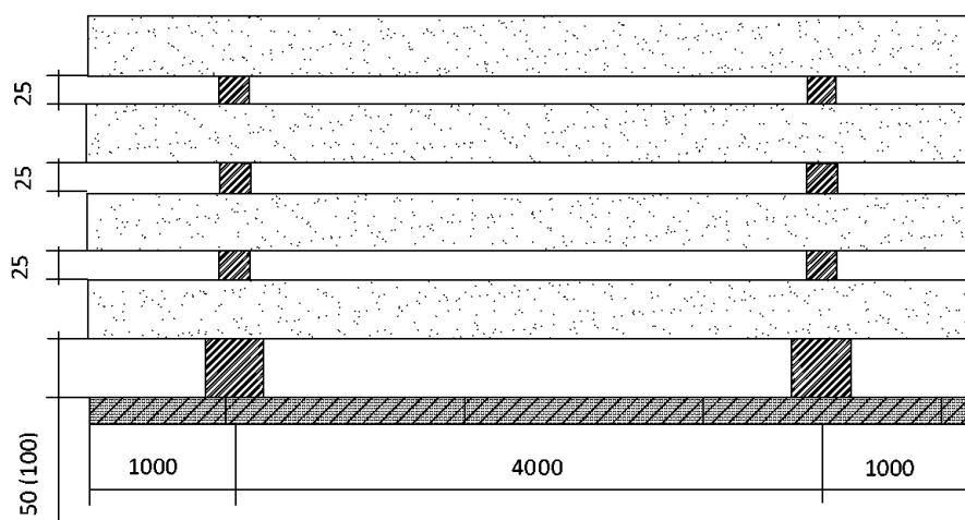
Рисунок 3 - Схема складирования плит
