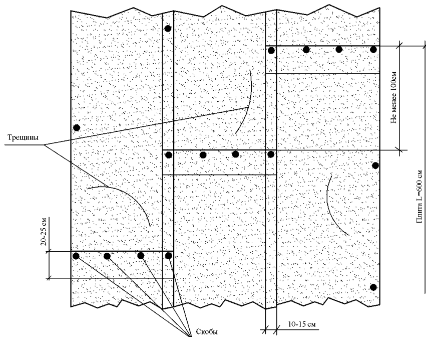
Рисунок 16 - Схема локальной укладки трещинопрерывающей (армирующей) прослойки в местах трещин и швов сборного цементобетонного покрытия
