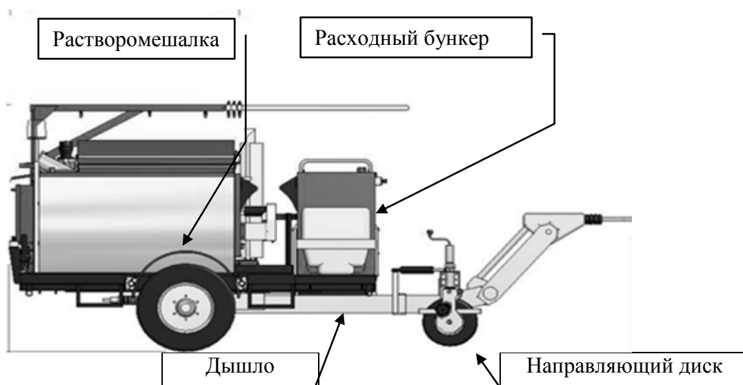
Рисунок 12 - Вариант конструкции заливщика шва
