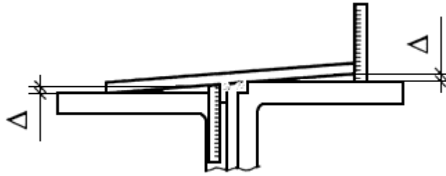
Рисунок И.18 – Измерение перекаса двумя угольниками и линейками
