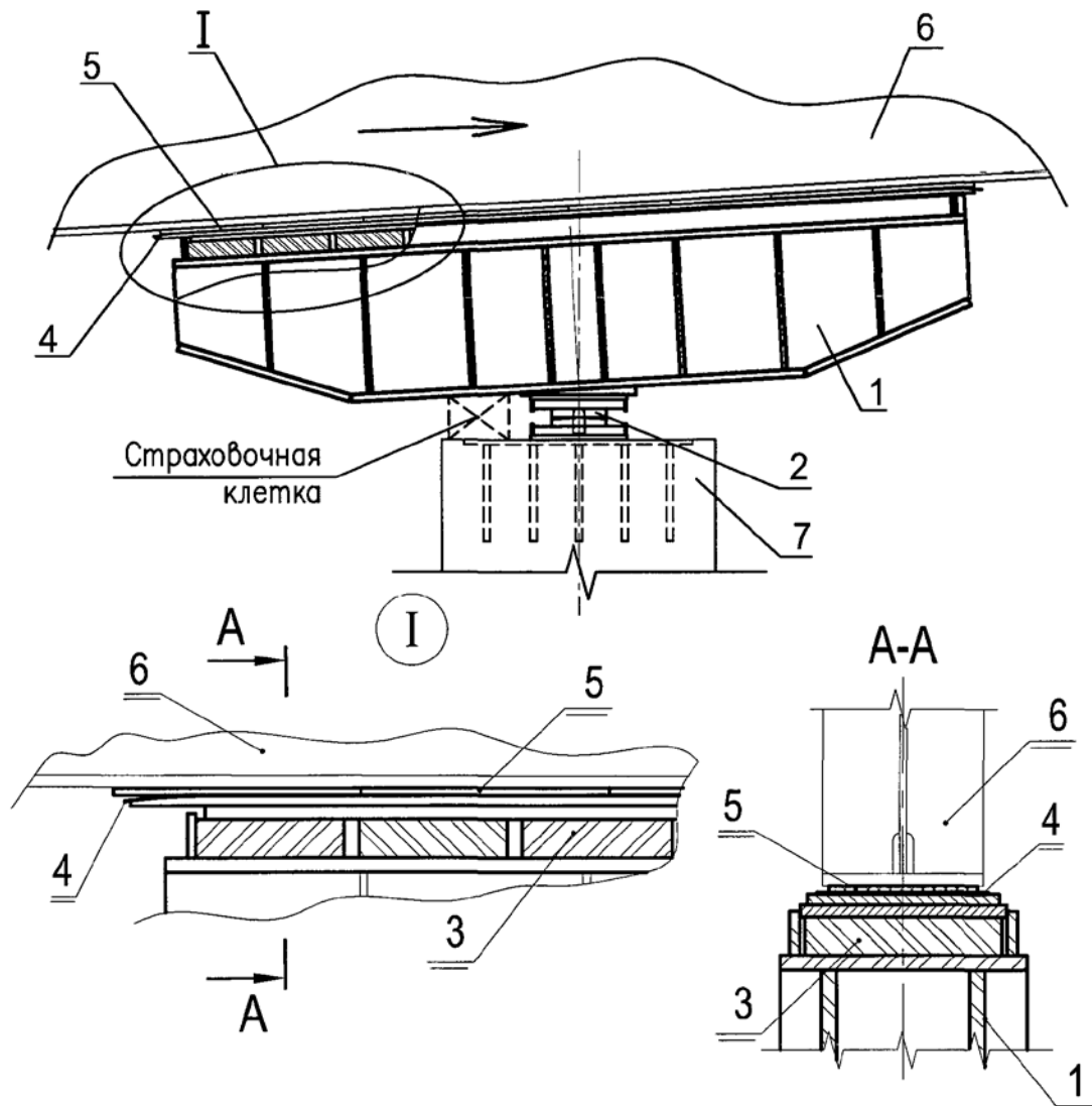
1 – накаточная (баланси́рная) балка; 2 – опорная часть (шарнир); 3 – резиновая прокладка; 4 – контртело (стальной полированный лист); 5 – полимерные прокладки (карточки скольжения); 6 – надвигаемая конструкция; 7 – подферменник опоры
