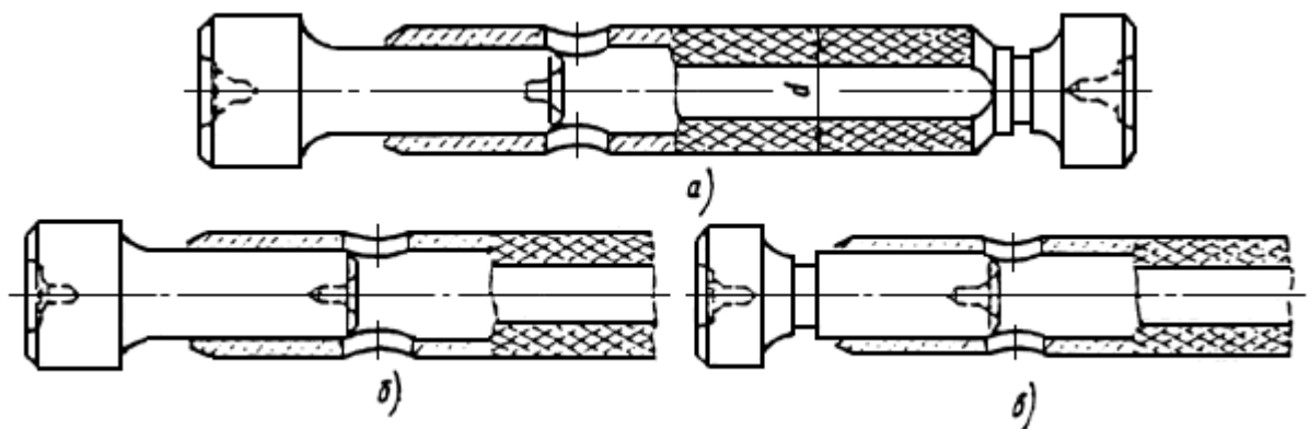
Рисунок И.14 – Калибры-пробки со вставками
